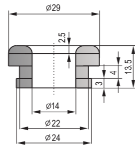
DT-039 EPDM密封墊圈 EPDM Sealing O-ring
