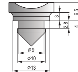
DT-044 EPDM緩衝門擋 EPDM door nail buffer
