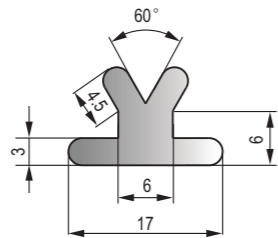
DFT-053 黑色EPDM海綿膠條 Black EPDM Sponge Strip
