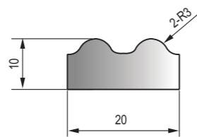
DFT-038 黑色EPDM海綿膠條 Black EPDM Sponge Strip
