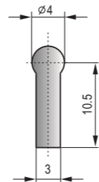
DFT-042 黑色EPDM海綿膠條 Black EPDM Sponge Strip
