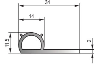
DFT-063 黑色EPDM密實膠條 Black EPDM Dense Strip
