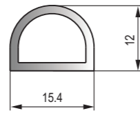
DFT-050 黑色EPDM海綿膠條 Black EPDM Sponge Strip
