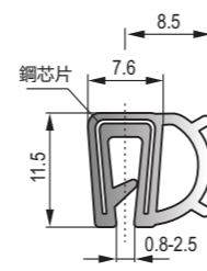
D-003 黑色EPDM鋼絲膠條 Black EPDM steel wire strip
