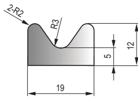
DFT-025 黑色EPDM海綿膠條 Black EPDM Sponge Strip
