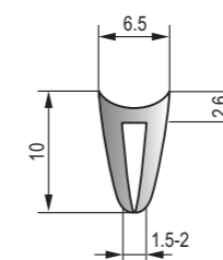
DFT-059 黑色EPDM密實膠條 Black EPDM Dense Strip
