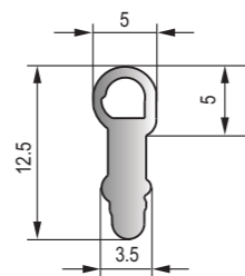
DFT-041 黑色EPDM海綿膠條 Black EPDM Sponge Strip
