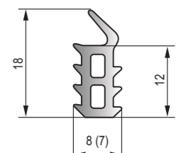
DFT-060 黑色EPDM密實膠條 Black EPDM Dense Strip
