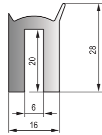
DFT-075 黑色EPDM密實膠條 Black EPDM Dense Strip
