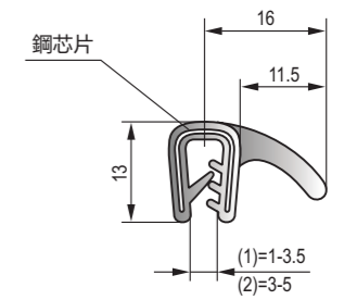
D-009 黑色EPDM鋼絲膠條 Black EPDM steel wire strip
