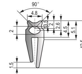
DFT-068 黑色EPDM密實膠條 Black EPDM Dense Strip
