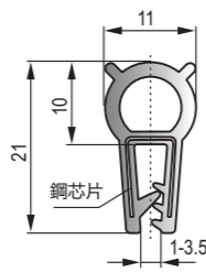
D-002 黑色EPDM鋼絲膠條 Black EPDM steel wire strip
