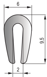
DFT-076 黑色EPDM密實膠條 Black EPDM Dense Strip
