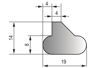
DFT-033 黑色EPDM海綿膠條 Black EPDM Sponge Strip
