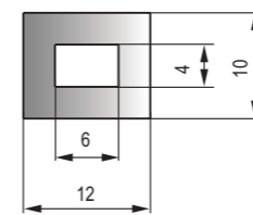
DFT-034 黑色EPDM海綿膠條 Black EPDM Sponge Strip
