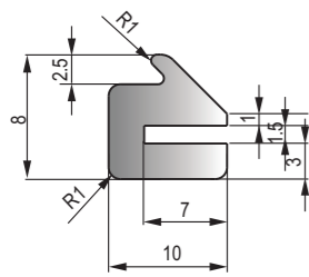
DFT-028 黑色EPDM海綿膠條 Black EPDM Sponge Strip
