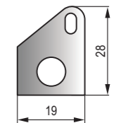
DFT-036 黑色EPDM海綿膠條 Black EPDM Sponge Strip
