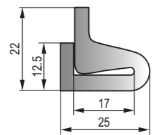
DFT-037 黑色EPDM海綿膠條 Black EPDM Sponge Strip
