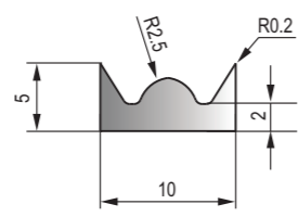
DFT-026 黑色EPDM海綿膠條 Black EPDM Sponge Strip
