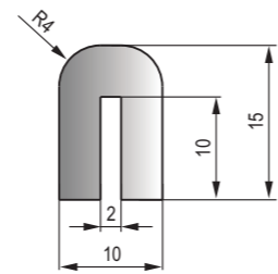
DFT-027 黑色EPDM海綿膠條 Black EPDM Sponge Strip
