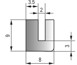
DFT-069 黑色EPDM密實膠條 Black EPDM Dense Strip
