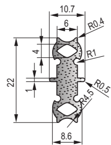
DFT-052 黑色EPDM海綿膠條 Black EPDM Sponge Strip
