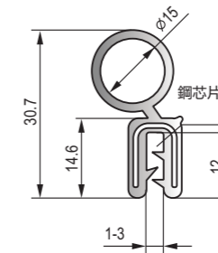
D-008 黑色EPDM鋼絲膠條 Black EPDM steel wire strip
