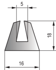
DFT-078 黑色EPDM密實膠條 Black EPDM Dense Strip
