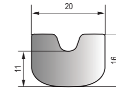
DFT-032 黑色EPDM海綿膠條 Black EPDM Sponge Strip
