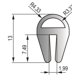
DFT-056 黑色EPDM密實膠條 Black EPDM Dense Strip
