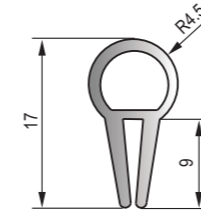
DFT-055 黑色EPDM密實膠條 Black EPDM Dense Strip
