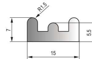
DFT-046 黑色EPDM海綿膠條 Black EPDM Sponge Strip
