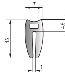
DFT-058 黑色EPDM密實膠條 Black EPDM Dense Strip
