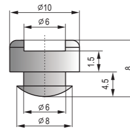
DT-043 EPDM緩衝門擋 EPDM door nail buffer
