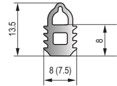
DFT-061 黑色EPDM密實膠條 Black EPDM Dense Strip
