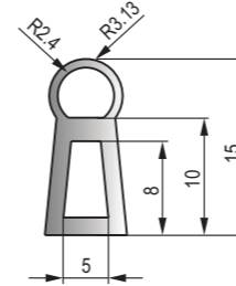
DFT-031 黑色EPDM海綿膠條 Black EPDM Sponge Strip
