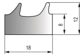
DFT-051 黑色EPDM海綿膠條 Black EPDM Sponge Strip
