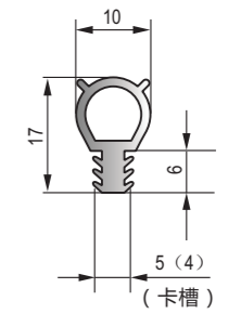
DFT-024 黑色EPDM密封條 Black EPDM sealing strip
