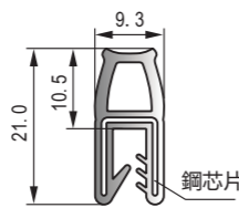
D-017 黑色EPDM鋼絲膠條 Black EPDM steel wire strip
