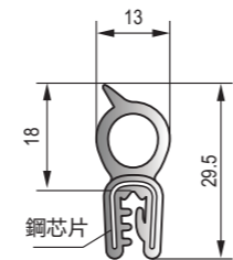
D-018 黑色EPDM鋼絲膠條 Black EPDM steel wire strip
