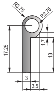
DFT-074 黑色EPDM密實膠條 Black EPDM Dense Strip
