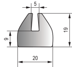
DFT-077 黑色EPDM密實膠條 Black EPDM Dense Strip
