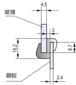
DFT-062 黑色EPDM密實膠條 Black EPDM Dense Strip
