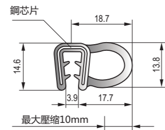
D-005 黑色EPDM鋼絲膠條 Black EPDM steel wire strip
