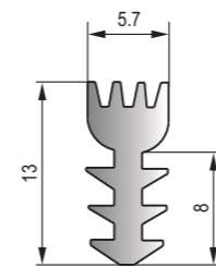
DFT-030 黑色EPDM海綿膠條 Black EPDM Sponge Strip
