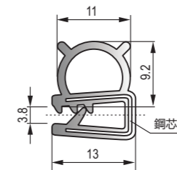
D-011 黑色EPDM鋼絲膠條 Black EPDM steel wire strip
