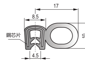
D-007 黑色EPDM鋼絲膠條 Black EPDM steel wire strip
