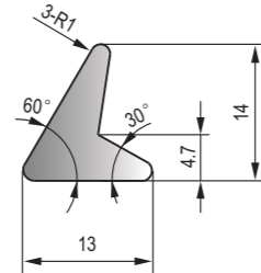
DFT-029 黑色EPDM海綿膠條 Black EPDM Sponge Strip
