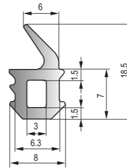
DFT-067 黑色EPDM密實膠條 Black EPDM Dense Strip
