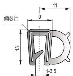
D-004 黑色EPDM鋼絲膠條 Black EPDM steel wire strip
