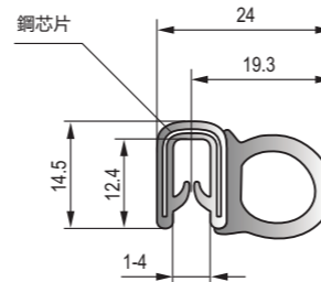
D-006 黑色EPDM鋼絲膠條 Black EPDM steel wire strip
