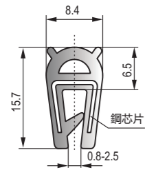
D-001 黑色EPDM鋼絲膠條 Black EPDM steel wire strip
