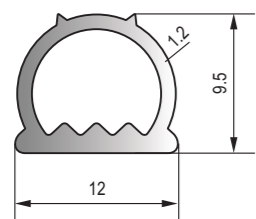
DFT-040 黑色EPDM海綿膠條 Black EPDM Sponge Strip
