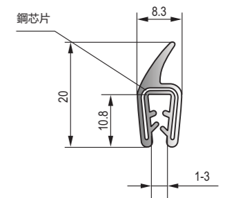
D-012 黑色EPDM鋼絲膠條 Black EPDM steel wire strip
