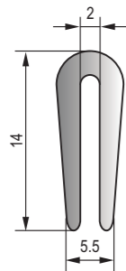
D-064 黑色EPDM密實膠條 Black EPDM Dense Strip
