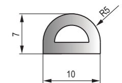
DFT-048 黑色EPDM海綿膠條 Black EPDM Sponge Strip
