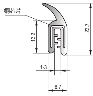
D-013 黑色EPDM鋼絲膠條 Black EPDM steel wire strip
