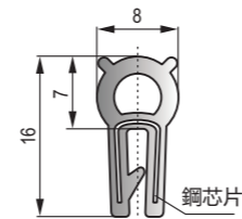
D-015 黑色EPDM鋼絲膠條 Black EPDM steel wire strip
