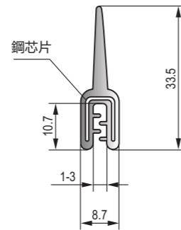
D-014 黑色EPDM鋼絲膠條 Black EPDM steel wire strip
