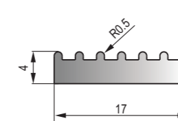
DFT-047 黑色EPDM海綿膠條 Black EPDM Sponge Strip
