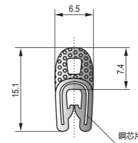
D-010 黑色EPDM鋼絲膠條 Black EPDM steel wire strip
