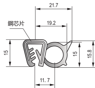
D-016 黑色EPDM鋼絲膠條 Black EPDM steel wire strip
